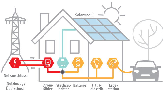
FUNKTIONSPRINZIP PHOTOVOLTAIK-ANLAGE
